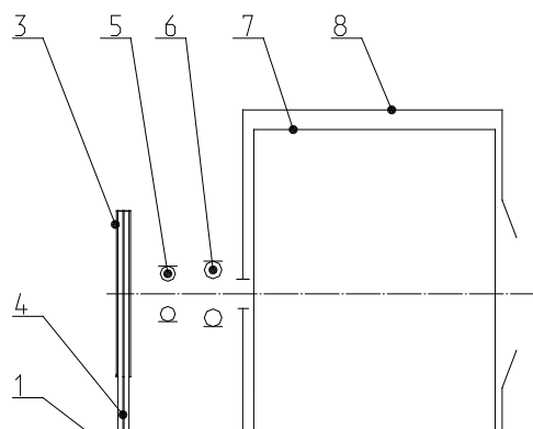
Кинематическая схема машины
