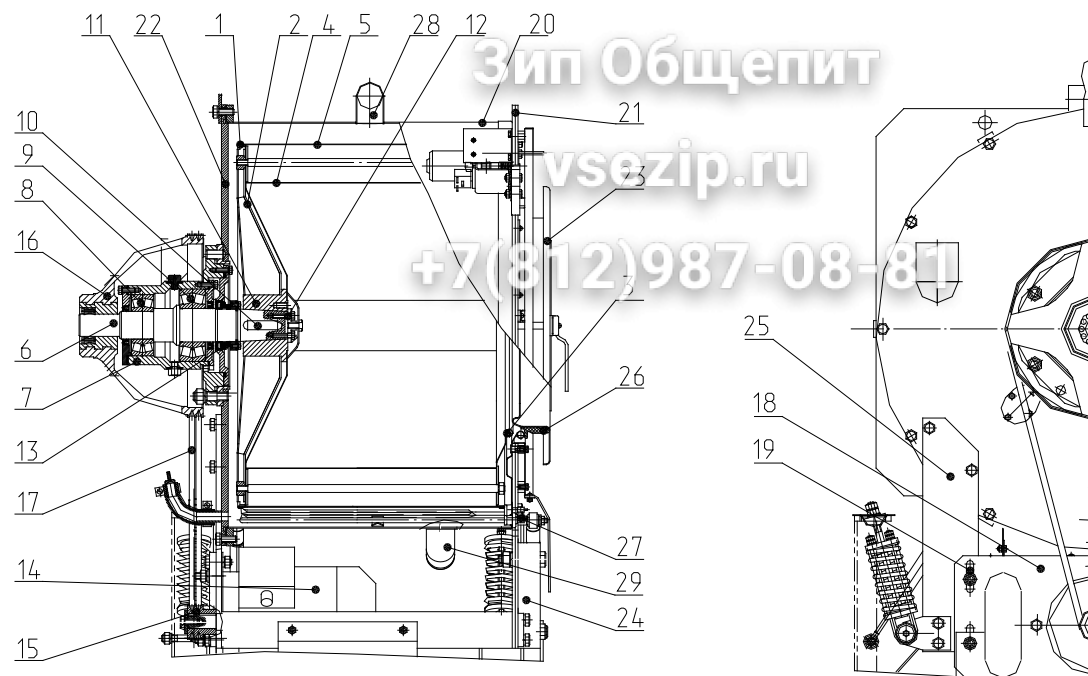
Рис.2 Блок барабанов
