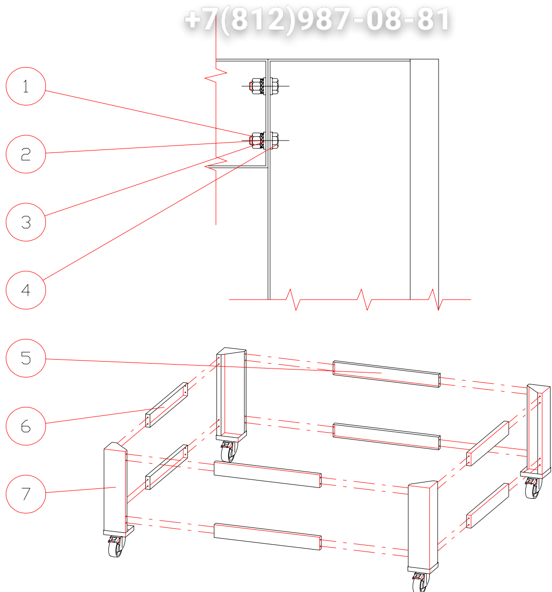
Abb. 10-9 Montage-Schema - Untergestell
