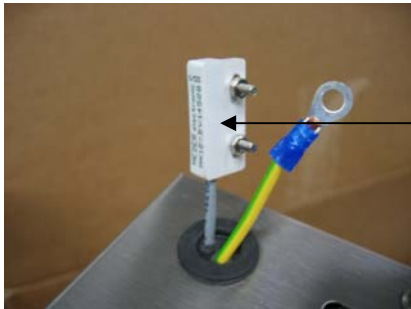
Magnetschalter / magnet switch, Teile-Nr. 3124228
